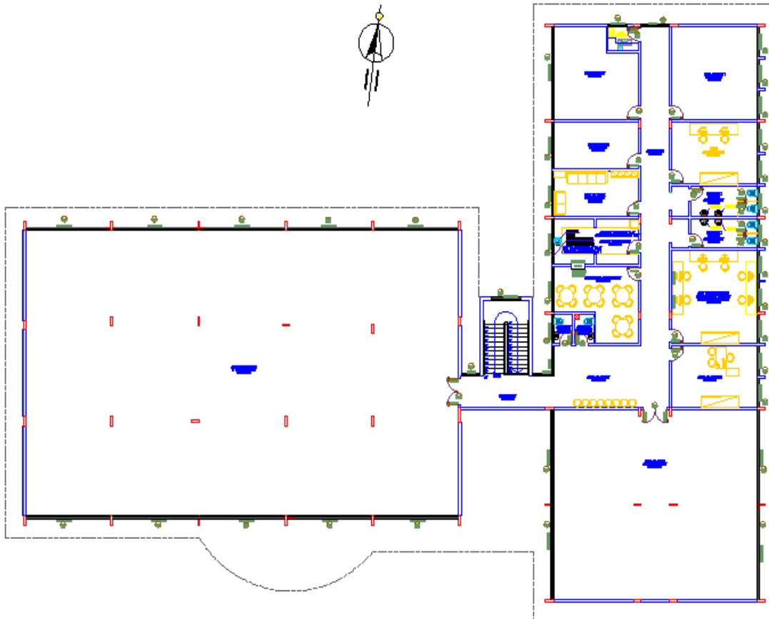
PLANTA BAIXA - PAVTO. SUPERIOR
